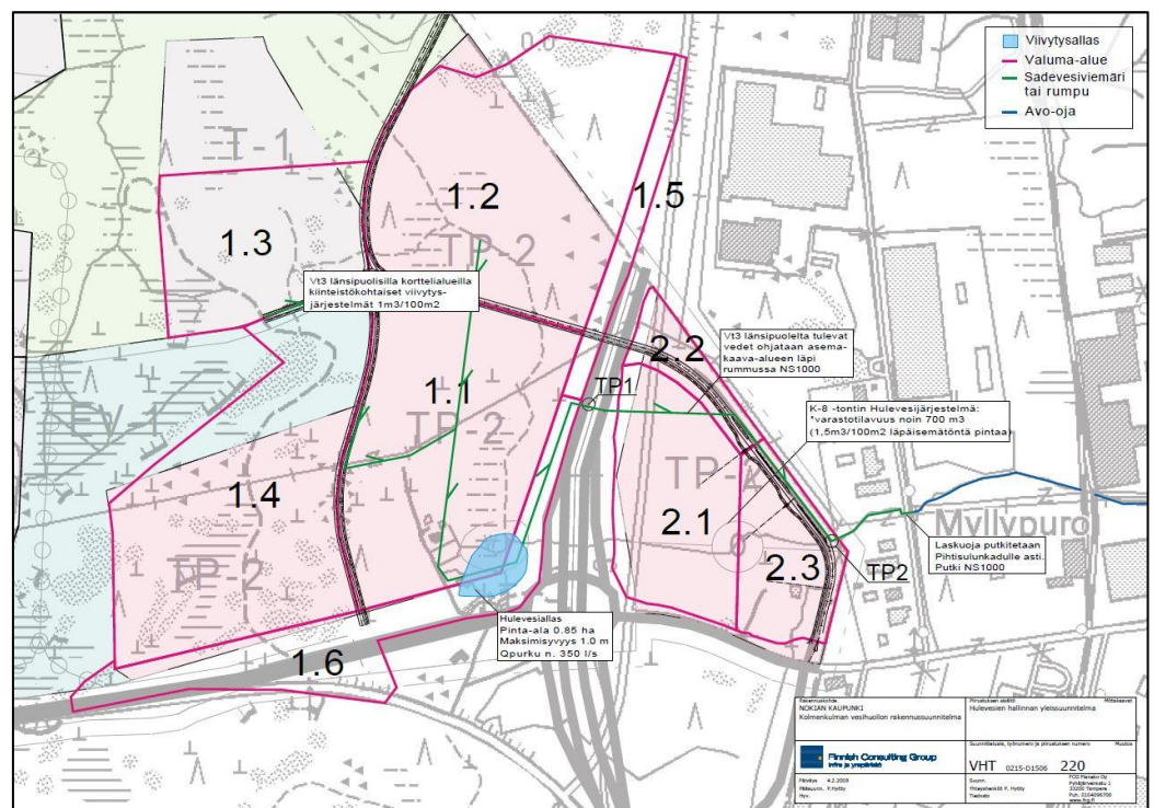
Kuva 9. Kolmenkulman itäosan hulevesien hallintasuunnitelmassa esitetyt hulevesien johtamis- ja käsittelyjärjestelyt. (FCG Planeko Oy 2009)
